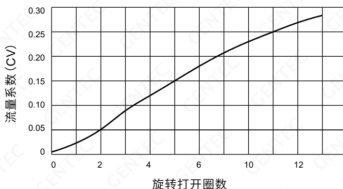
旋转打开时的流量系数
